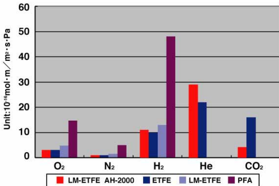
LM-ETFE AH-2000のガス透過率データ Gas permeation of LM-ETFE AH-2000
